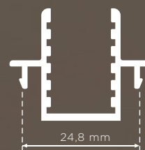
Aluminijski reduktor Značajke: za širinu žlijeba krila od 24-25mm
