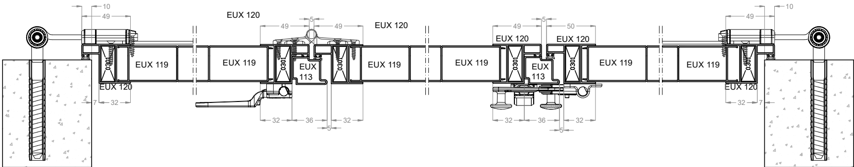
Otvaranje na preklop TP
